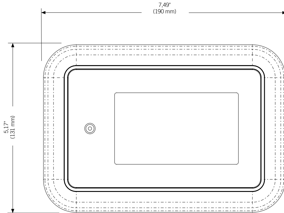
Front - Ansicht
